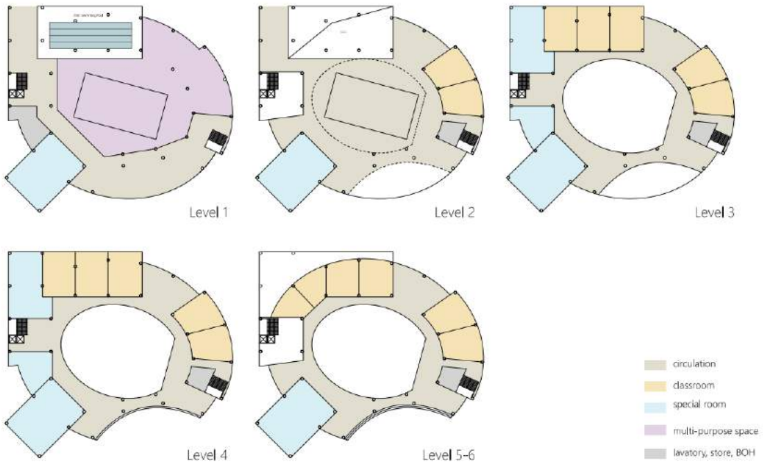
초등학교평면도
